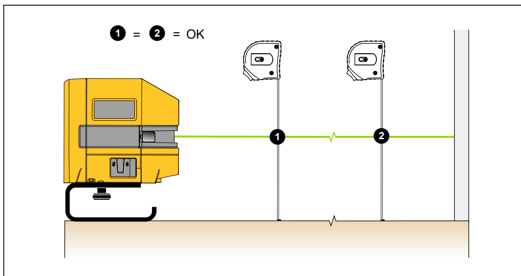
Obrázek 3. Zaměření stávajícího objektu
