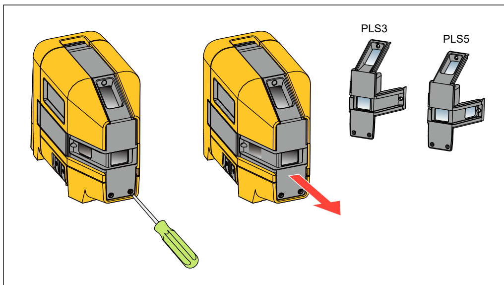
Obrázek 9. Nahrazení výměnného tělesa s optikou
