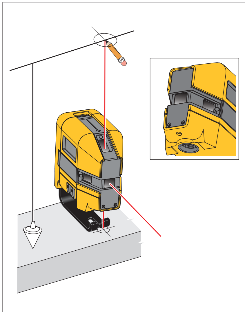
그림 4. 새 수직 표시
