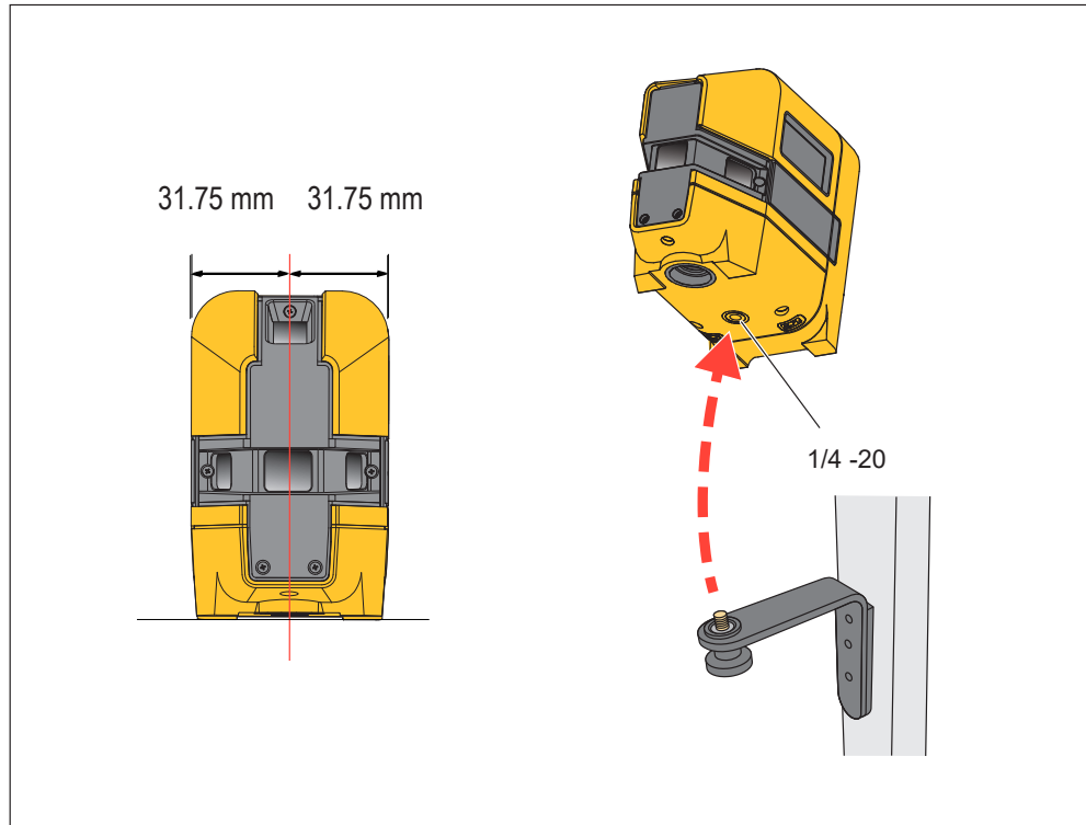
그림 1. 중심점 및 액세서리 마운트
