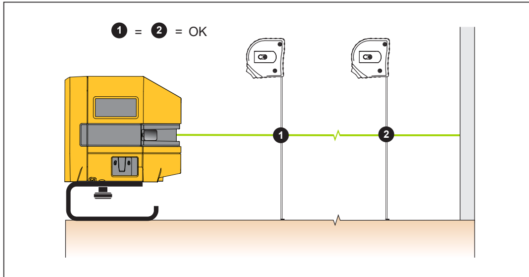
그림 3. 기존 항목 정렬
