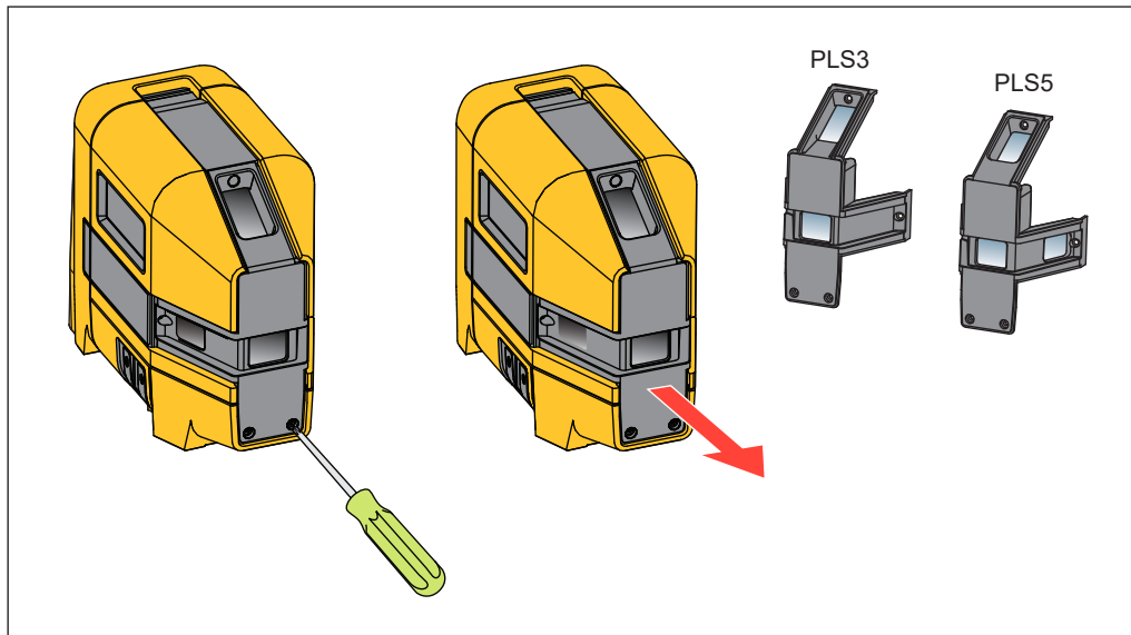
그림 9. 하우징 유리 insert 교체
