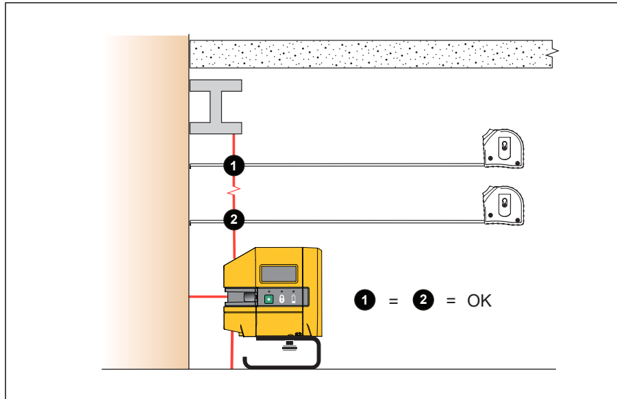
그림 5. 기존 항목 수직 점검
