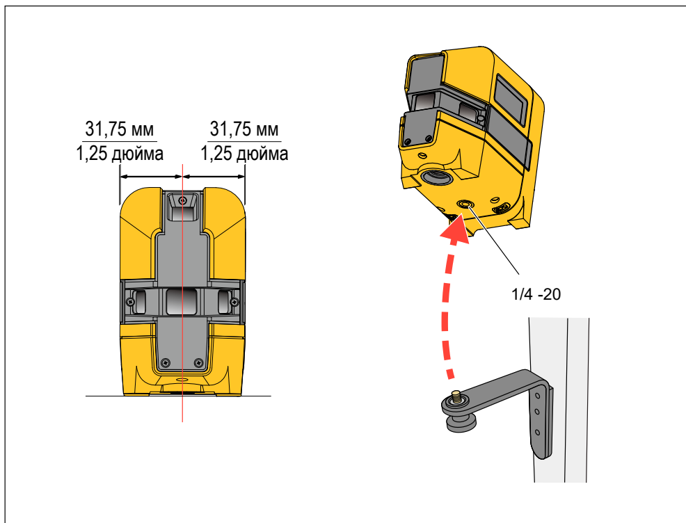
Рисунок 1. Центральная точка и дополнительное крепление
