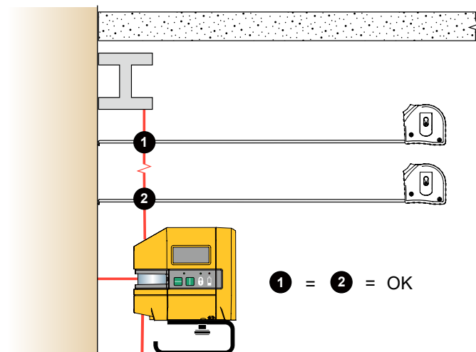
Obrázek 6. Ověření kolmosti stávajícího objektu
