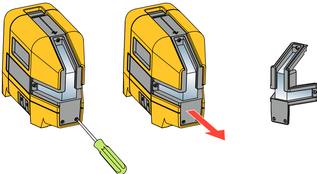
Obrázek 11. Nahrazení výměnného tělesa s optikou
