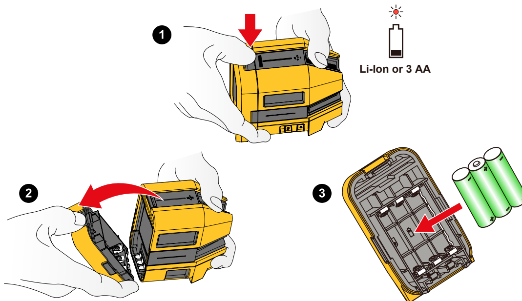
10. ábra Elemcsere
