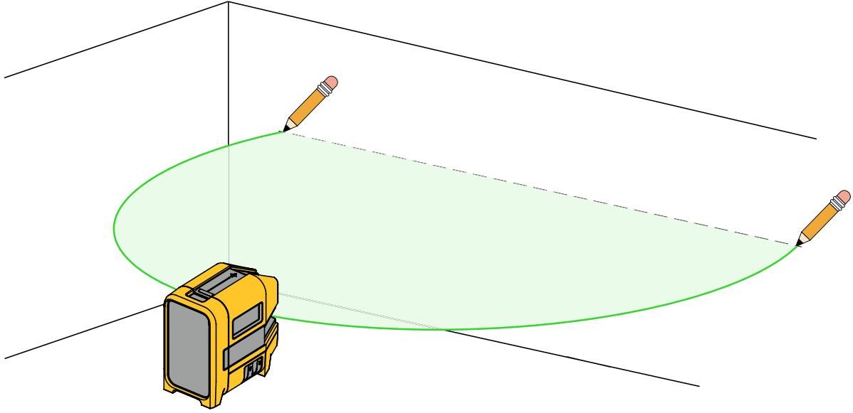
Şekil 2. Yeni Yatay ya da Diyagonal Hizalama
