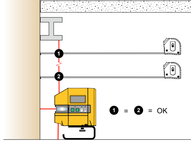
Şekil 6. Mevcut Öge Çekül Kontrolü
