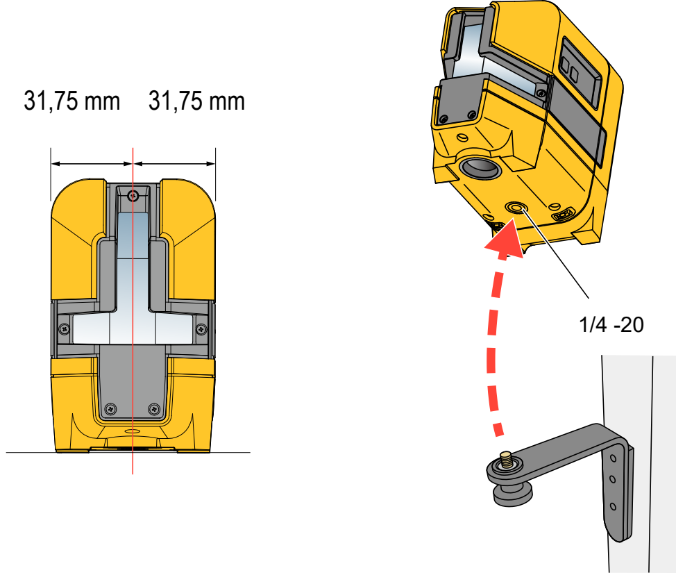
Şekil 1. Merkez Noktası ve Aksesuar Montajı
