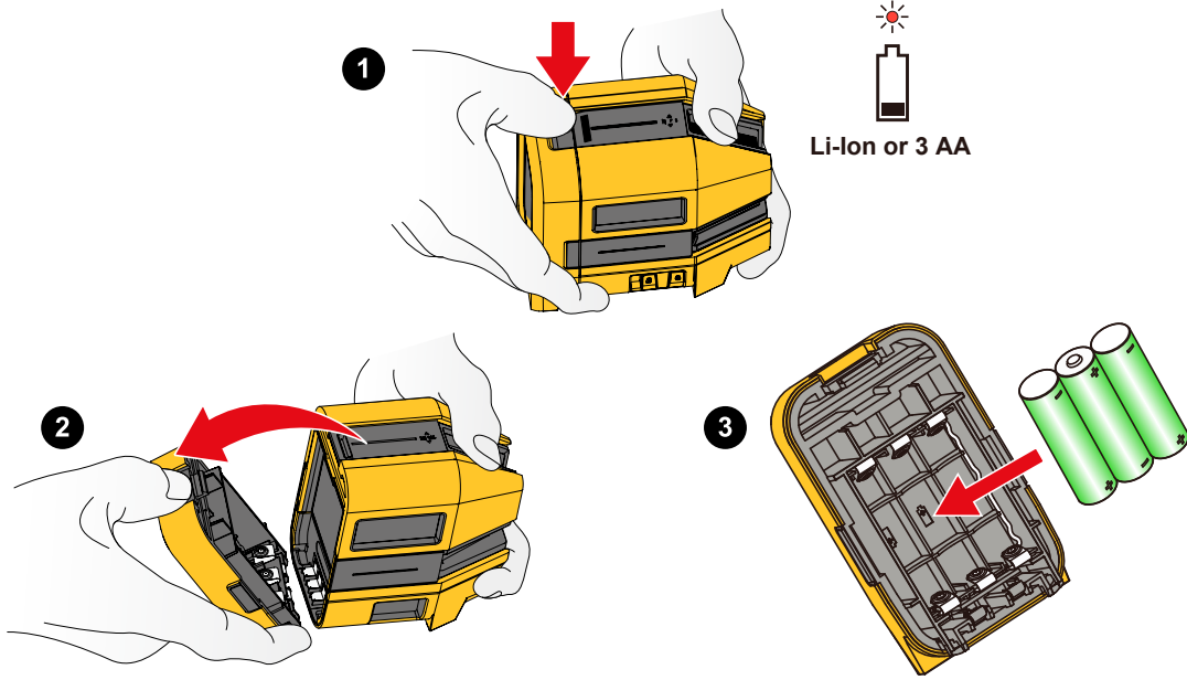
Şekil 10. Pil Değişimi
