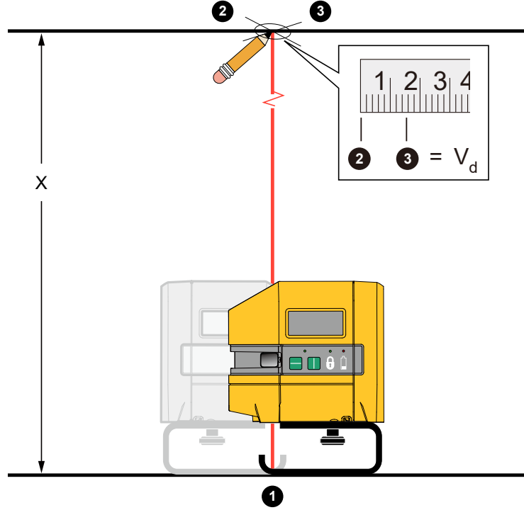
Şekil 9. Çekül Hassaslığı
